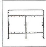
Geländer ZE links und rechts: Maße: 2040x1560x260 mm Gewicht: 40 kg (2 Stück)
